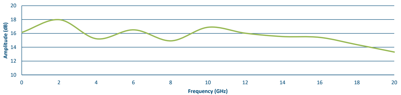
OP1dB
