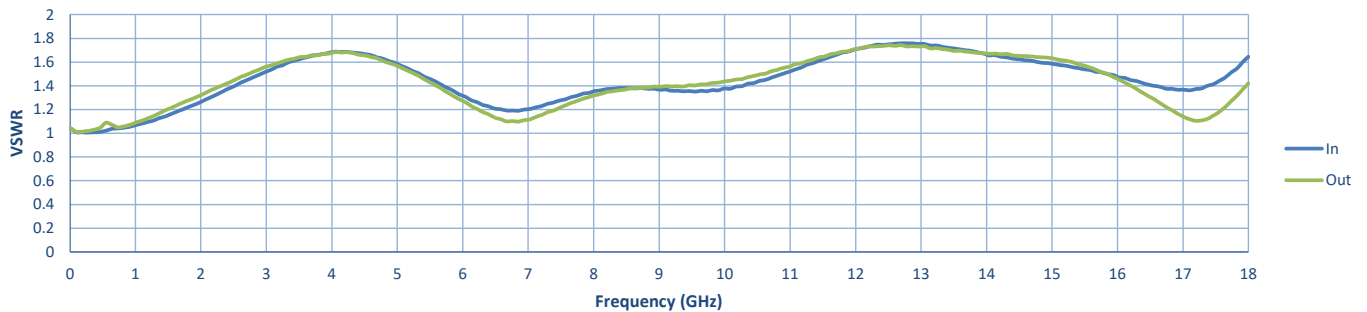
VSWR
